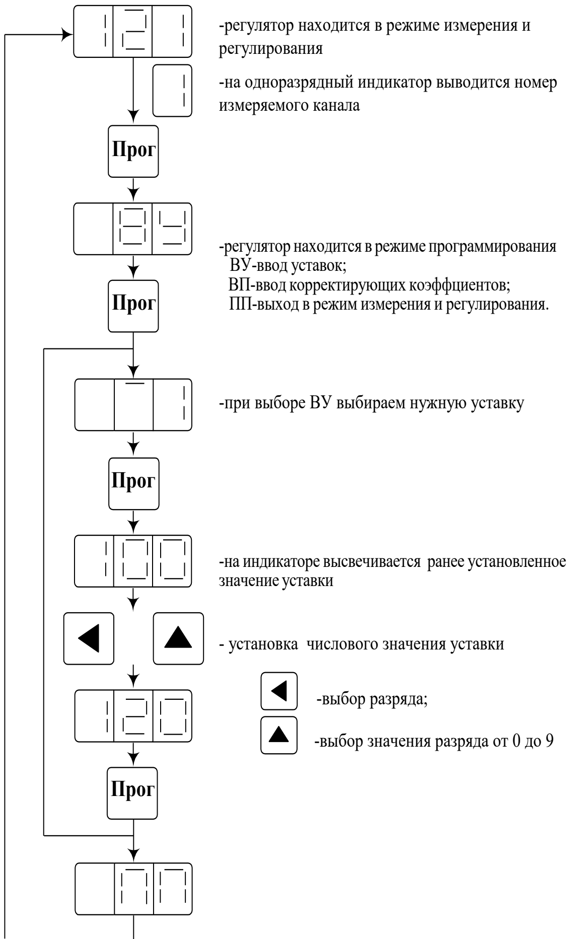
Рисунок 9 – Алгоритм работы регулятора в режиме ввода уставок
